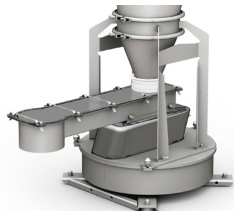
V200 Vibrationsdosierer in Hygienic Design (HD) mit geschlossener Rinne
