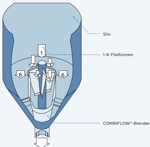
Silokonusmischer CFB
