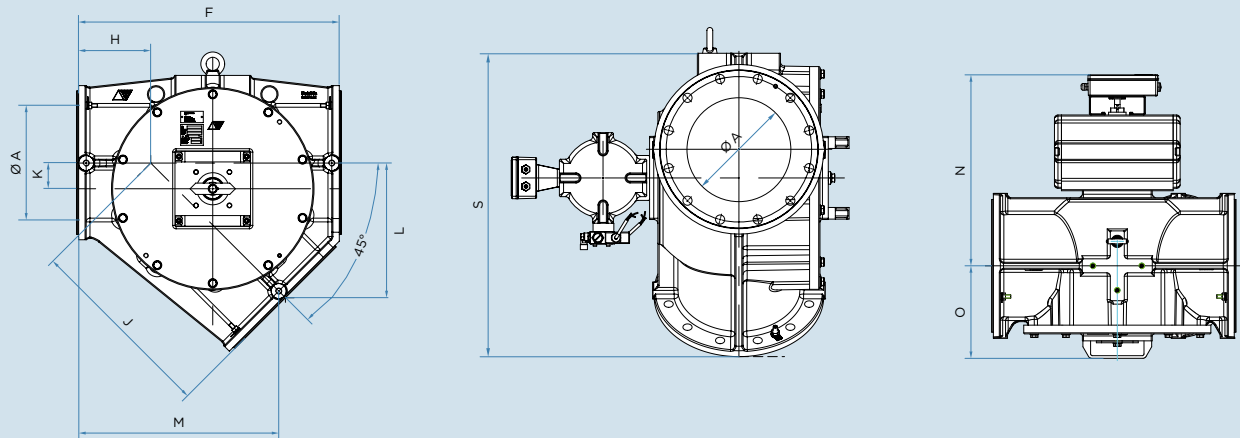
Darstellung mit Antrieb links
