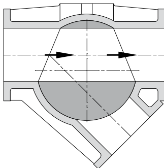
Gerader Durchgang
