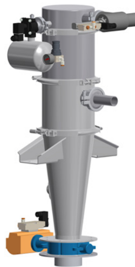
P10 Abscheider mit 100 mm [4 in] Drehklappenventil
