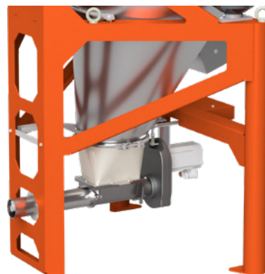
ProRate PLUS-L Dosierer mit Vertikalauslauf (oben) und Horizontalauslauf (unten).
