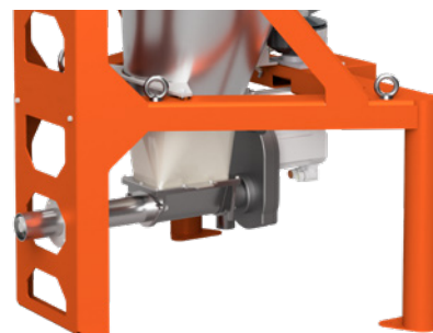
ProRate PLUS-M Dosierer mit Vertikalauslauf (oben) und Horizontalauslauf (unten).
